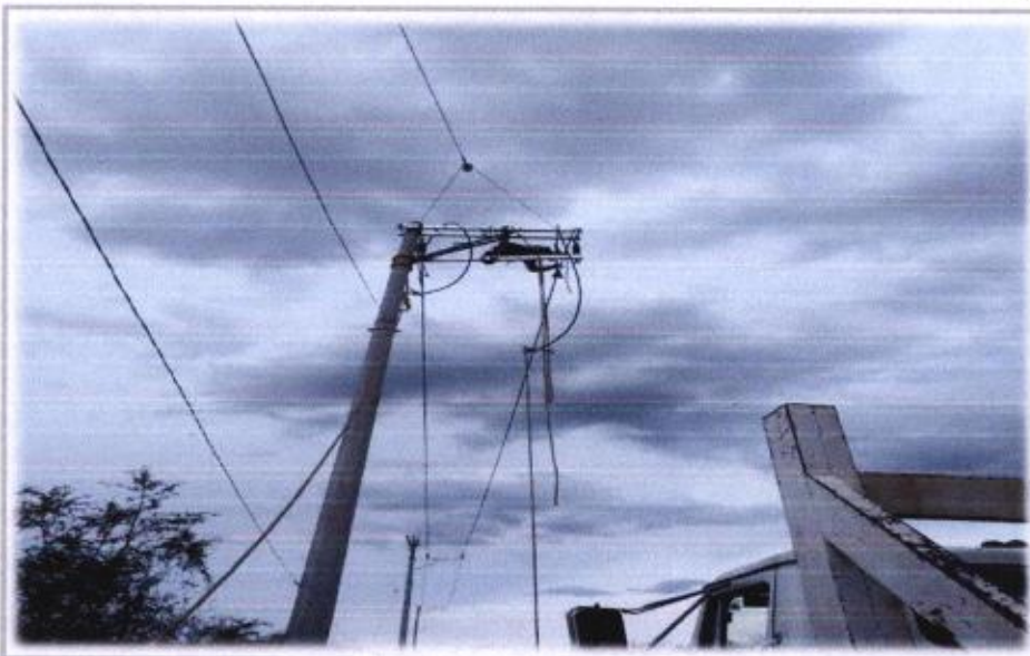
ESTRUCTURA VS3N.
